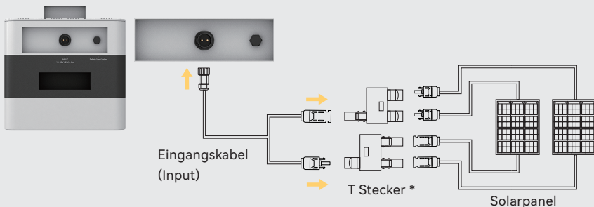
Diagramm - Parallelschaltung:
